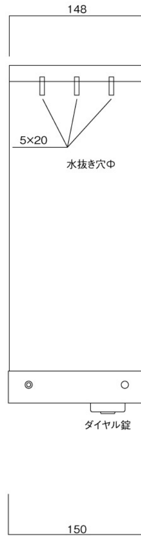
底面図
