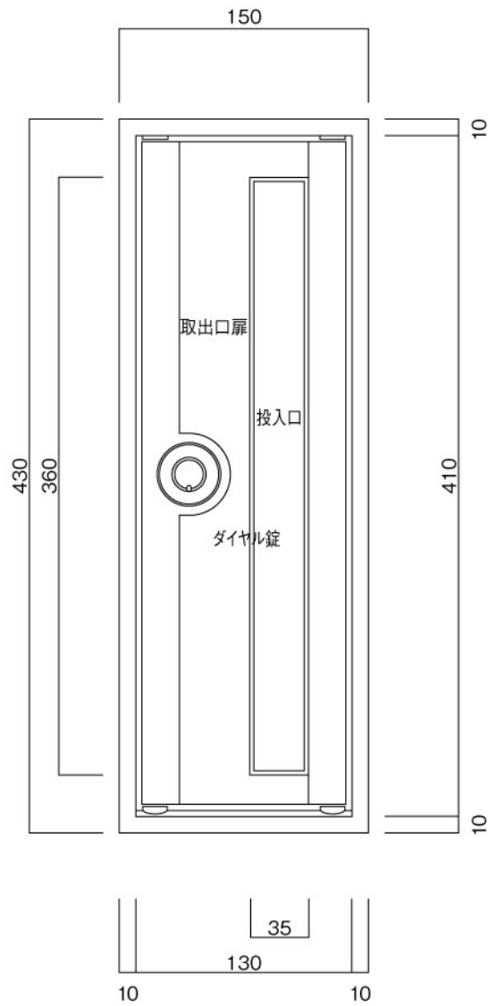
正面図
