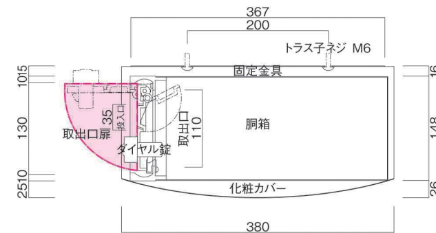
横断面図
