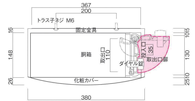
横断面図
