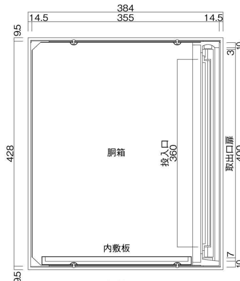
縦断面図
