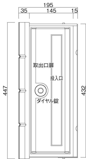
右側面図
