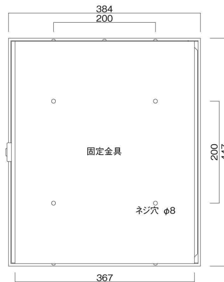
裏面図
