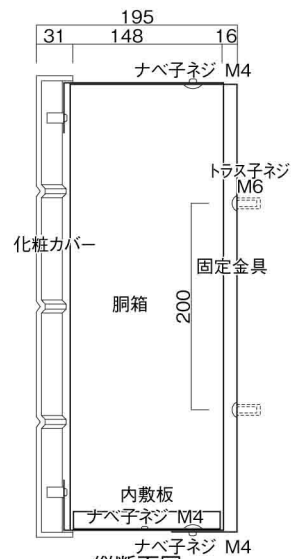
縦断面図
