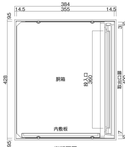
縦断面図
