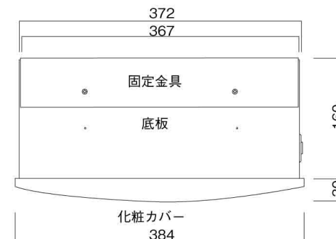
底面図
