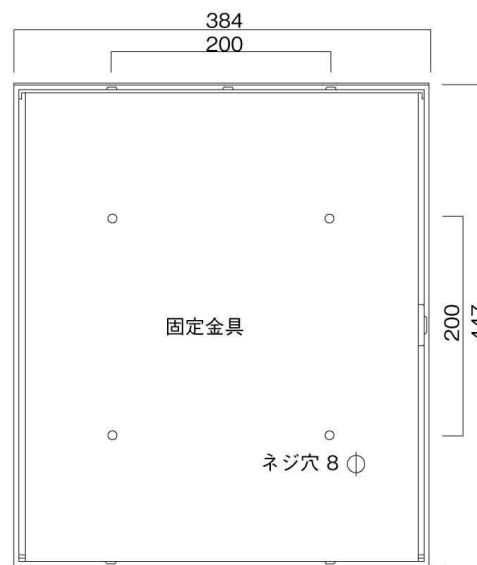
裏面図
