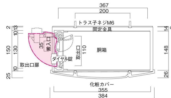
横断面図
