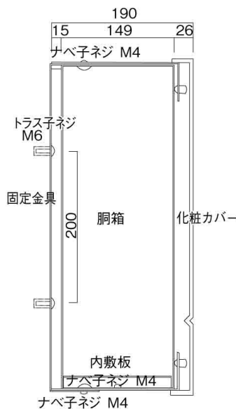
縦断面図
