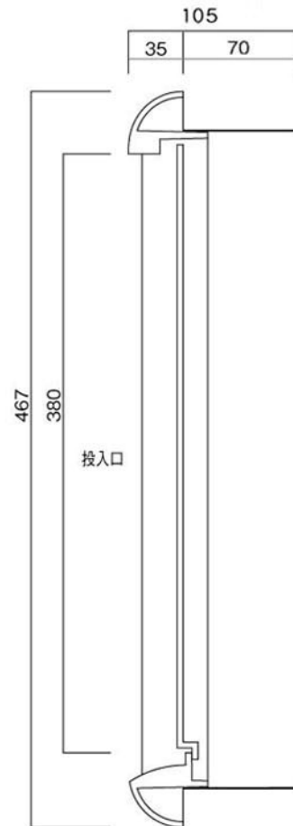
縦断面図
